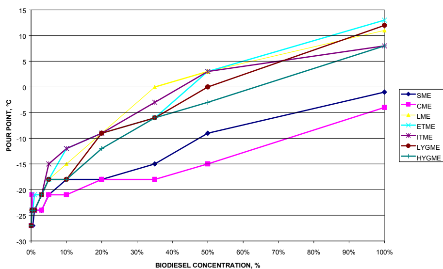
Figure 11. Biodiesel/diesel blend pour point test results
